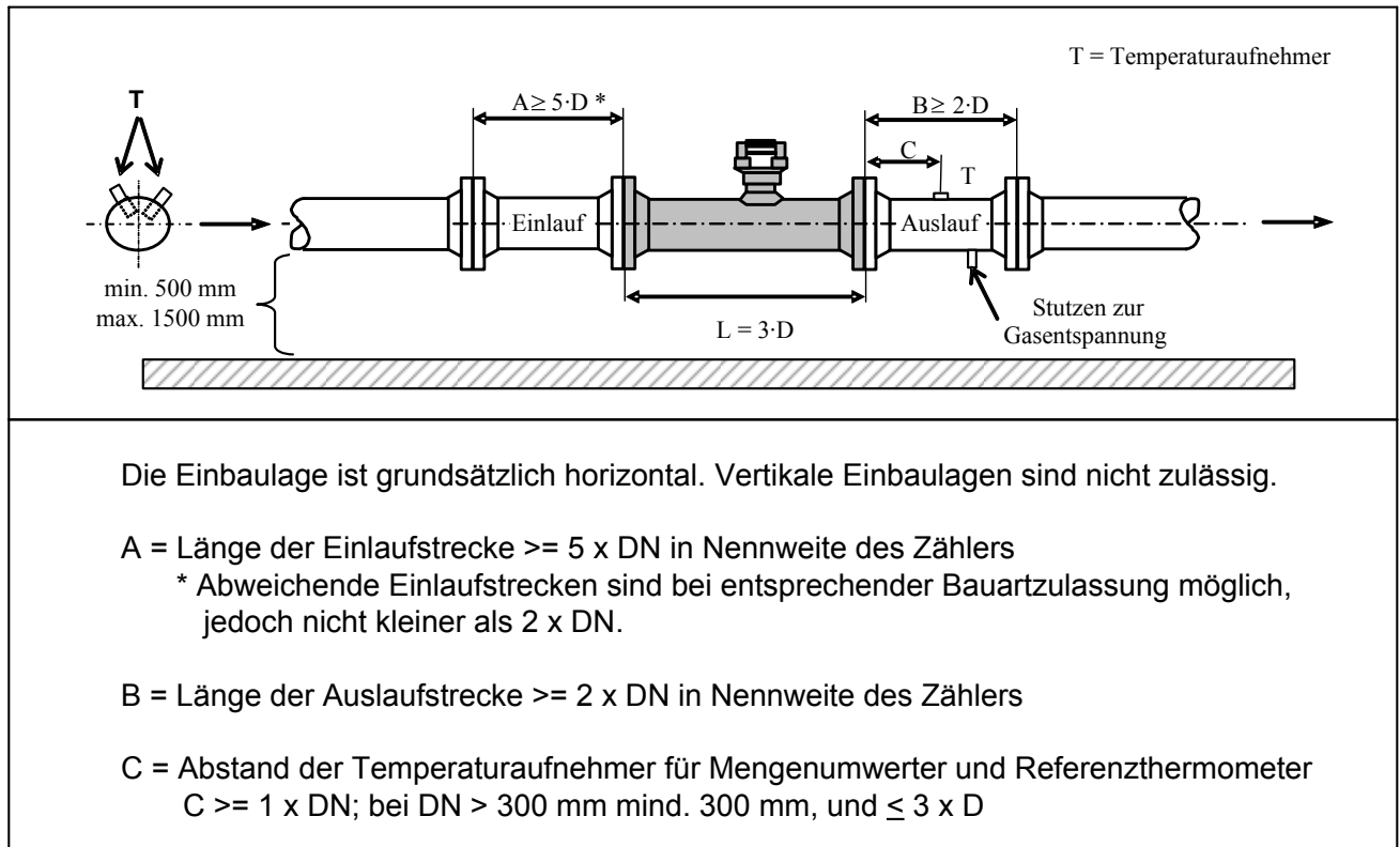
Bild 5: Installationsvorschrift für TRZ
