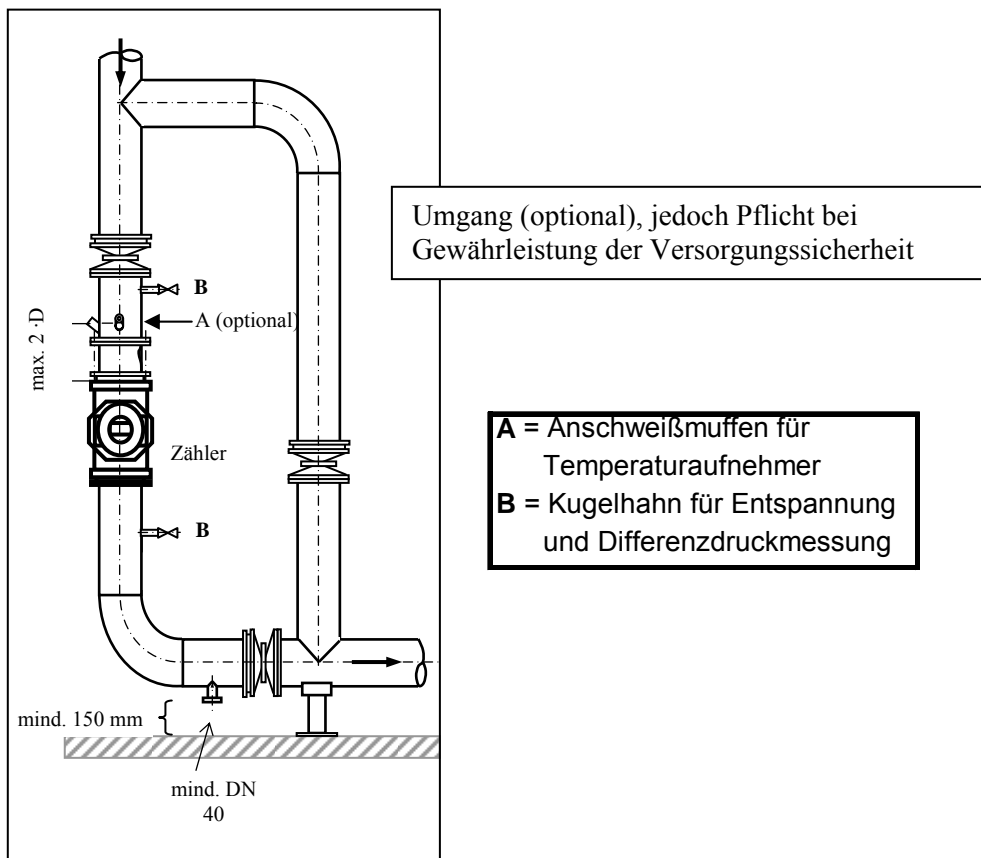
Bild 3: Messstelle (Zählergröße q_B \text{ max} < 650 \text{ m}^3/\text{h} ) mit optionaler Umgangsleitung
